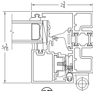
2B JAMB W/HINGE
