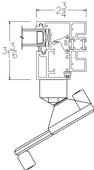
④ OPERABLE JAMB W/CRANK
