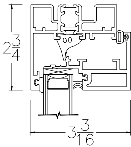
④ OPERABLE JAMB W/CRANK
