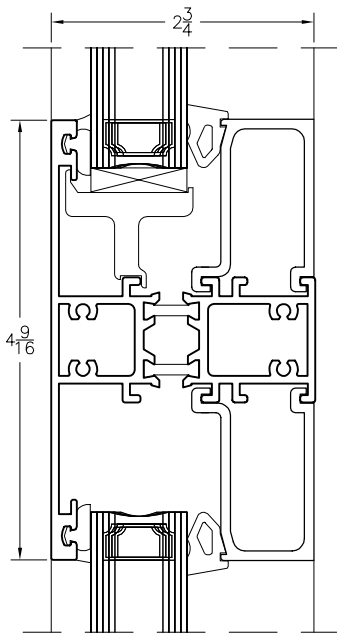
⑦ FX/FX TRANSOM
