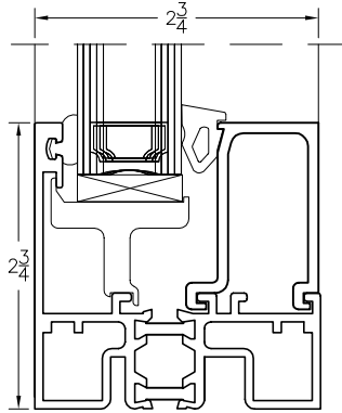
⑤ FX ● SILL
